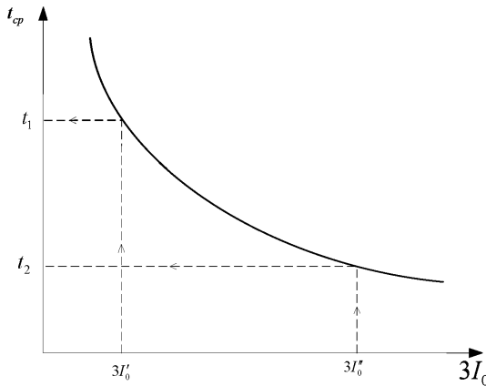
Рисунок В.4 – Обратно-зависимая характеристика выдержки времени t_{C3} защиты от тока ОЗЗ
