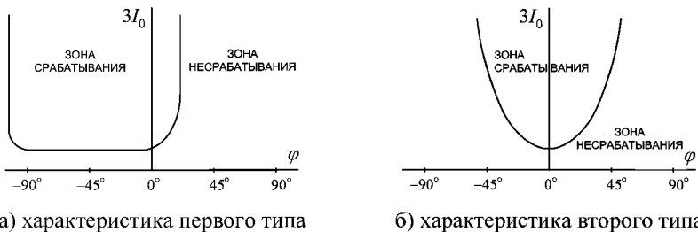
Рисунок В.2 – Фазовые характеристики направленных токовых защит от ОЗЗ, применяемых в сети с резистивным заземлением нейтрали
