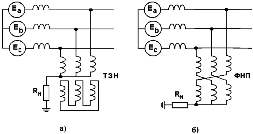
Рисунок 8.1 – Схемы включения резисторов в сети 35 кВ: а) в нейтраль обмотки высокого напряжения со схемой соединения обмоток Y0/Δ; б) в нейтраль фильтра нулевой последовательности
