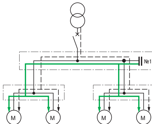
Рис. L14. Централизованная компенсация
