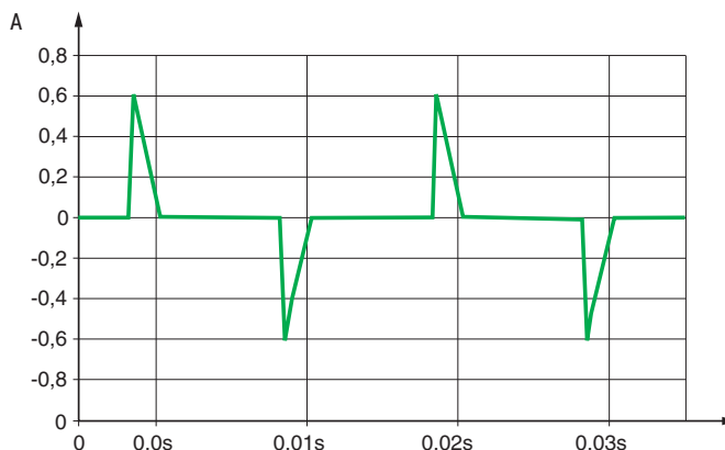
Рис. М7. Типовая форма кривой тока компактной люминесцентной лампы
