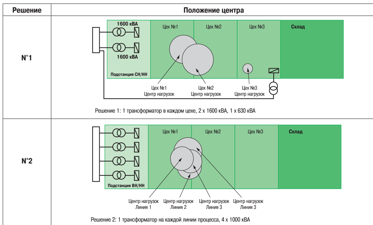
Рис. D30. Пример определения положения центра нагрузки
