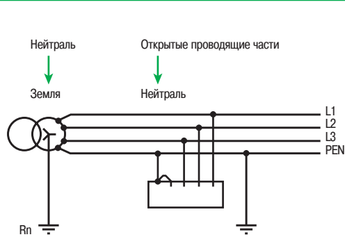
Рис. E4. Система TN-C
