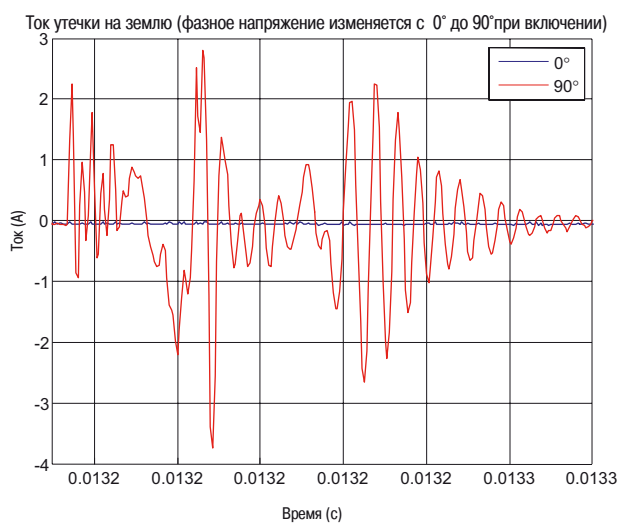
Рис. N53. Результат испытания утечки тока замыкания на землю
