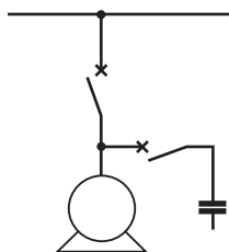
Рис. L27. Подсоединение блока конденсаторов к двигателю
