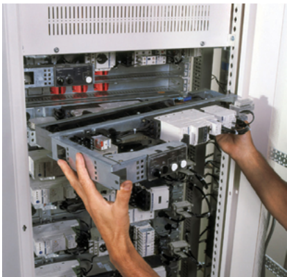
Рис. E31. РУ с вытчными функциональными блоками
