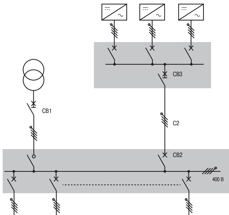
Рис. P35. Расположение автоматических выключателей
