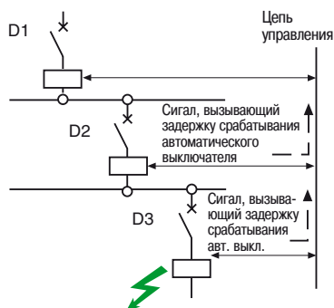
Рис. H55. Логическая селективность
