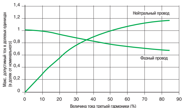
Рис. G23b. Максимальные допустимые токи (о.е.) в шинопровode в зависимости от уровня 3-й гармоники
