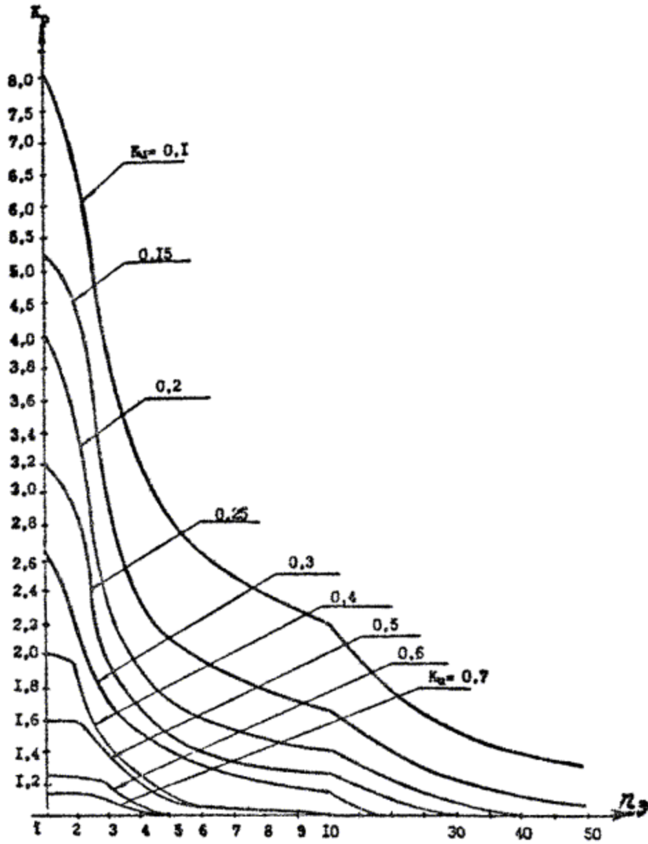
Кривые коэффициента расчетных нагрузок K_p для различных коэффициентов использования K_i в зависимости от n (для постоянной времени нагрева T_0=10 мин)
