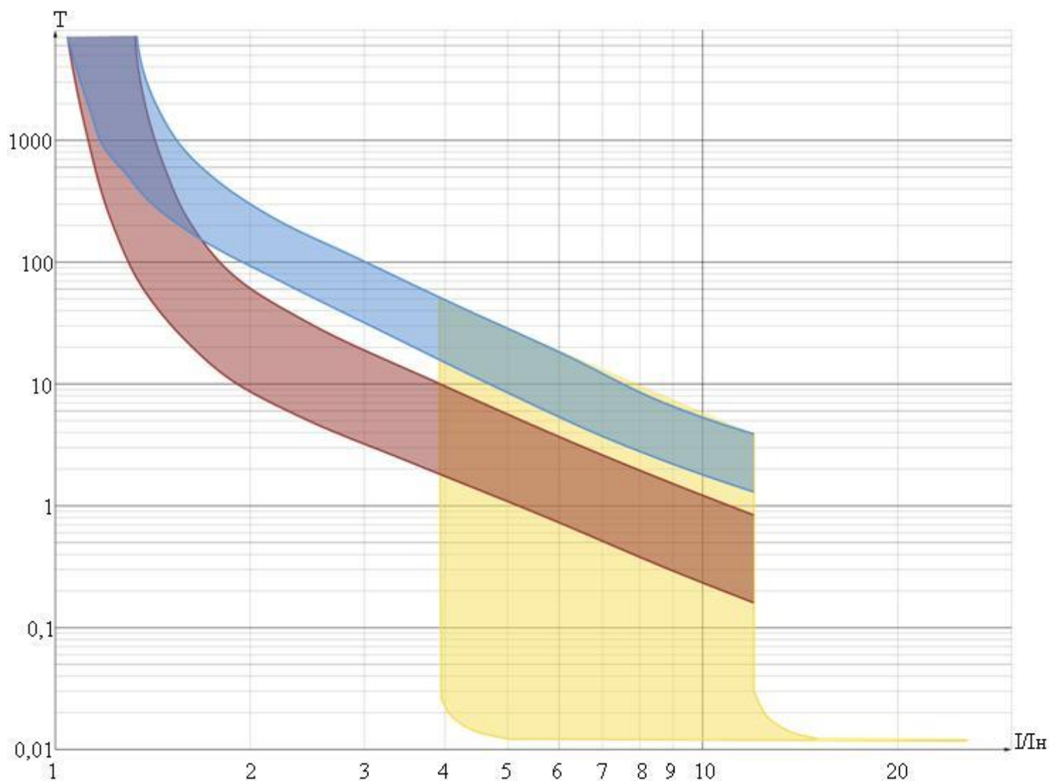
Рисунок Ж.8 - Время-токовые характеристики выключателя BA57-35 для номинальных токов тепловых максимальных расцепителей тока 100, 125 А
