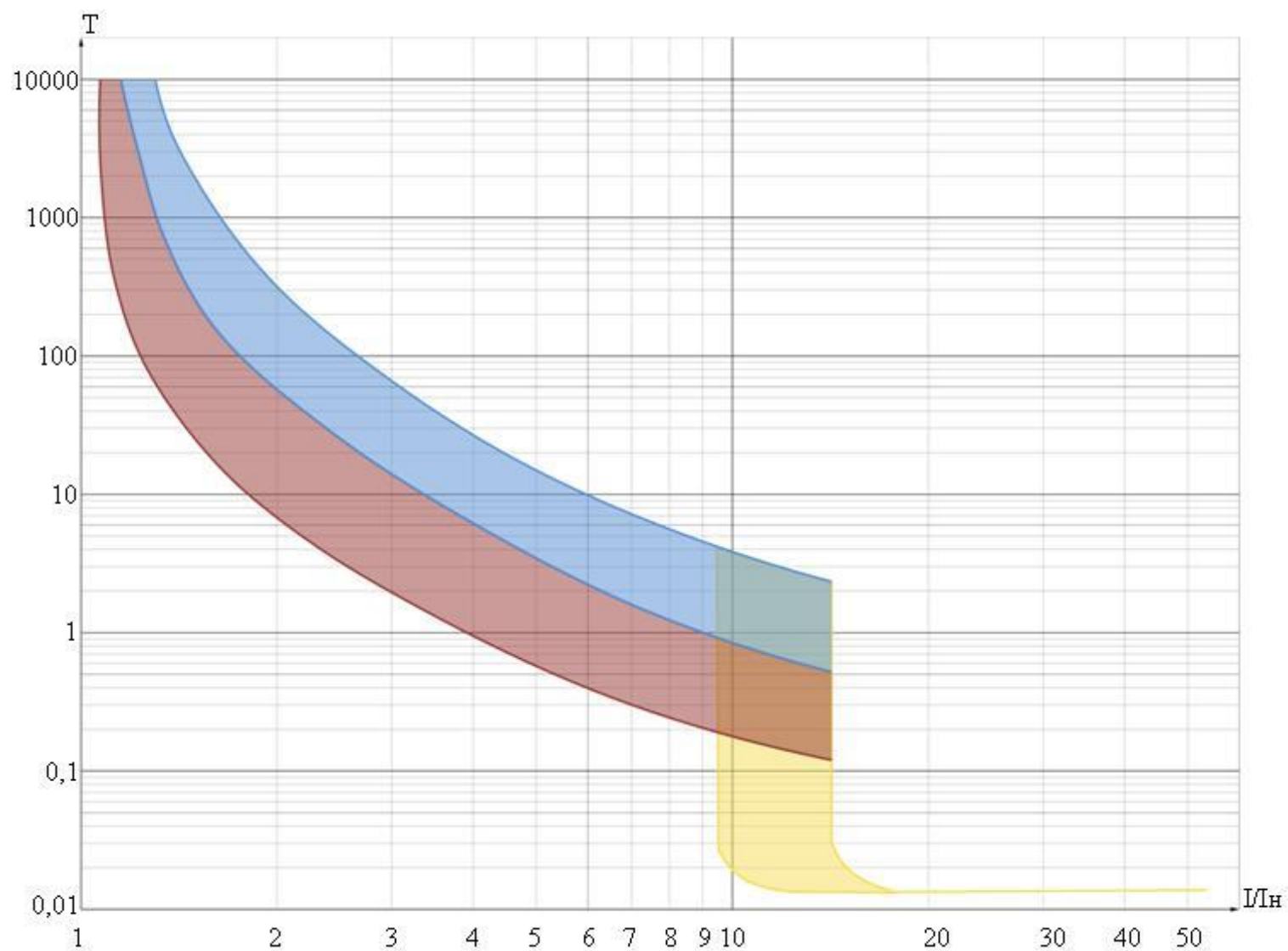
Рисунок Ж.4 - Время-токовые характеристики выключателя ВА04-36
