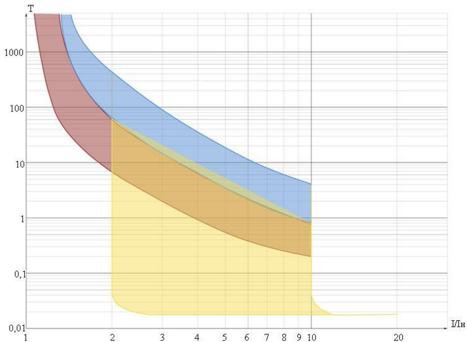
Рисунок Ж.10 - Время-токовые характеристики выключателя BA57-39
