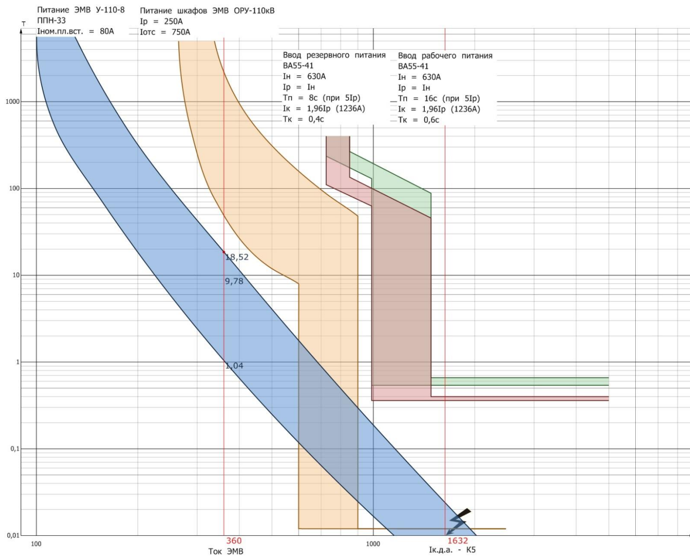
Рисунок Ж.2 - Карта селективности защитных аппаратов (с измененными характеристиками расцепителей)
