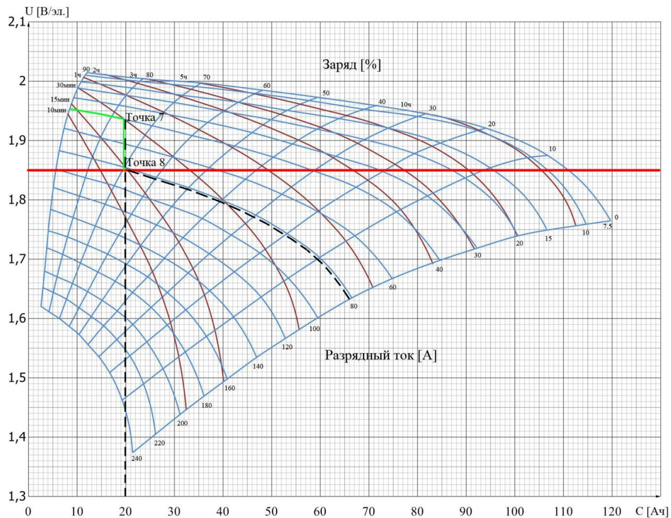
Рисунок В.6 - Разрядные характеристики пластины GroE 100 (расчет по шагу 4)
