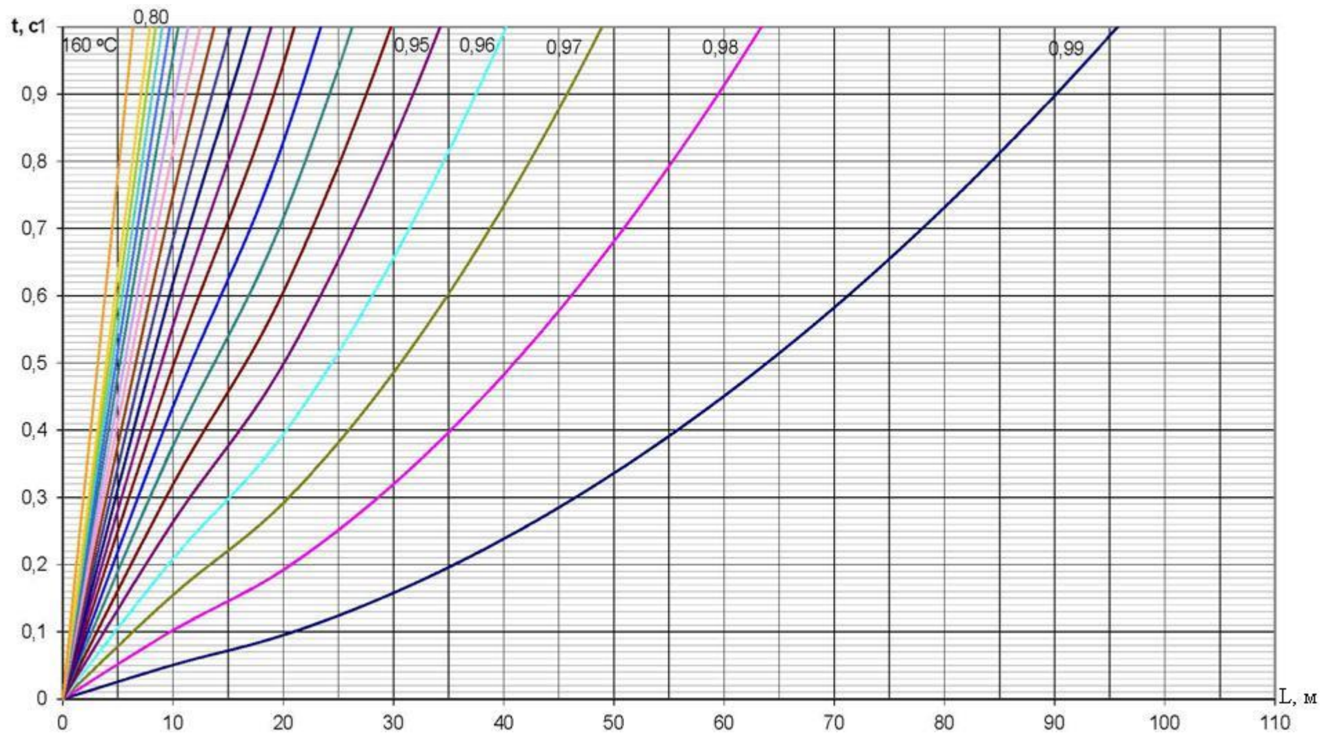
Рисунок Д.10 - Зависимость величины конечного тока (дугового средневекторного в % от начального) от времени протекания и длины кабеля S=16\text{мм}^2
