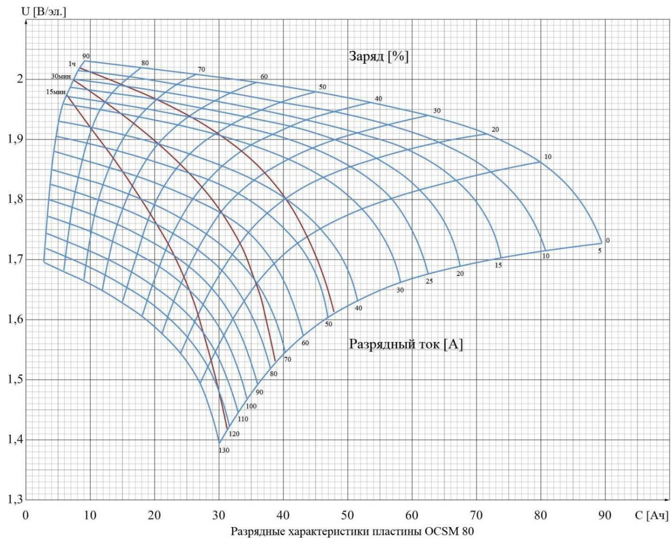
Рисунок В.13 - Разрядные характеристики пластины OCSM 80
