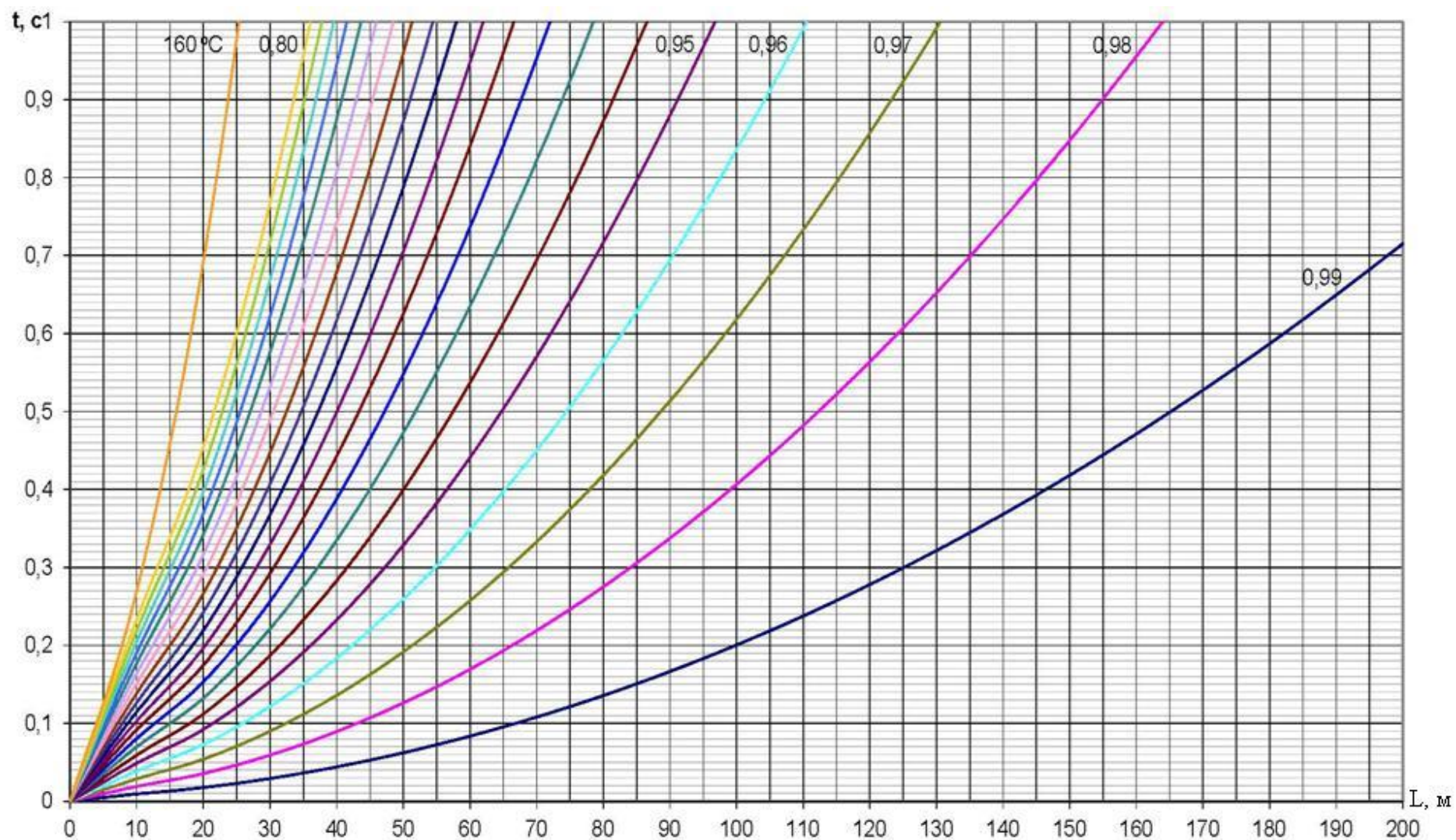
Рисунок Д.5 - Зависимость величины конечного тока (металлического в % от начального) от времени протекания и длины кабеля S=6\text{мм}^2
