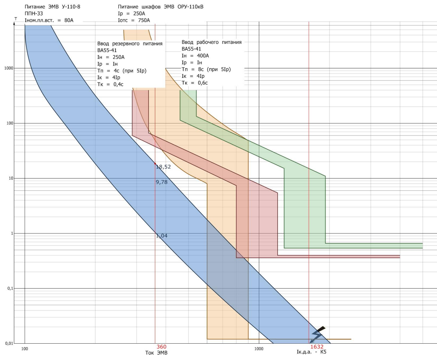
Рисунок Ж.1 - Карта селективности защитных аппаратов (предварительная)
