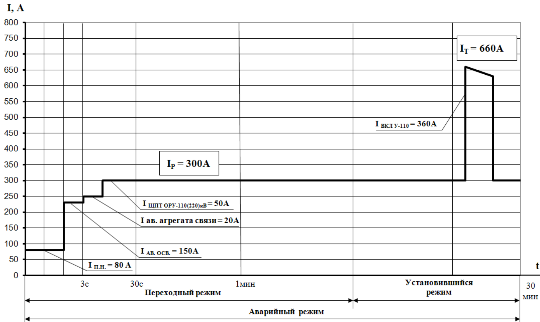
Рисунок В.1 - График нагрузки АВ при питании потребителей ЩПТ-1,2 в режиме аварийного получасового разряда
