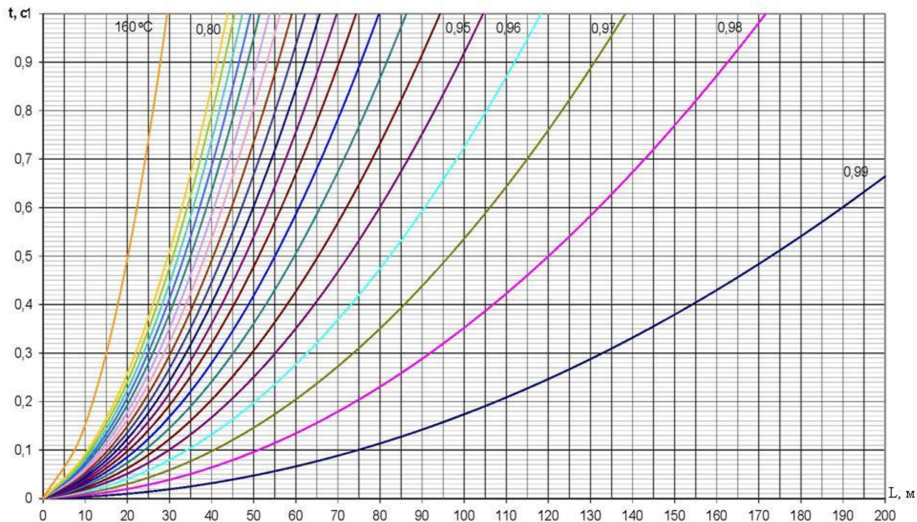
Рисунок Д.3 - Зависимость величины конечного тока (металлического в % от начального) от времени протекания и длины кабеля S=4\text{мм}^2
