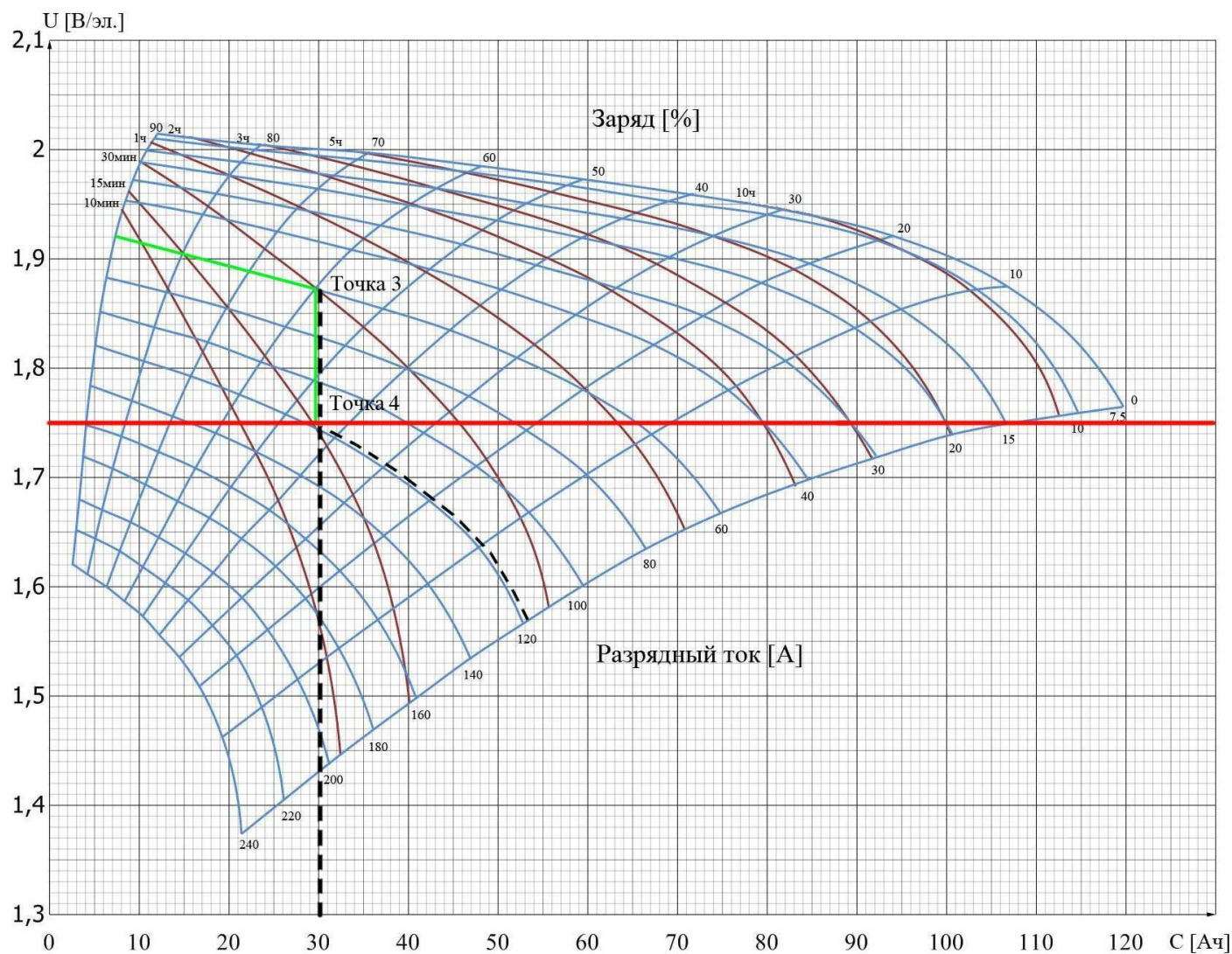
Рисунок В.3 - Разрядные характеристики пластины GdO 100 (расчет по шагу 2)
