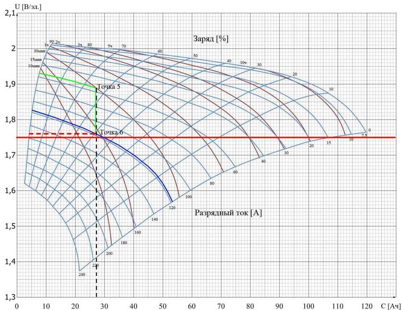
Рисунок В.4 - Разрядные характеристики пластины GrogE 100 (расчет по шагу 3)
