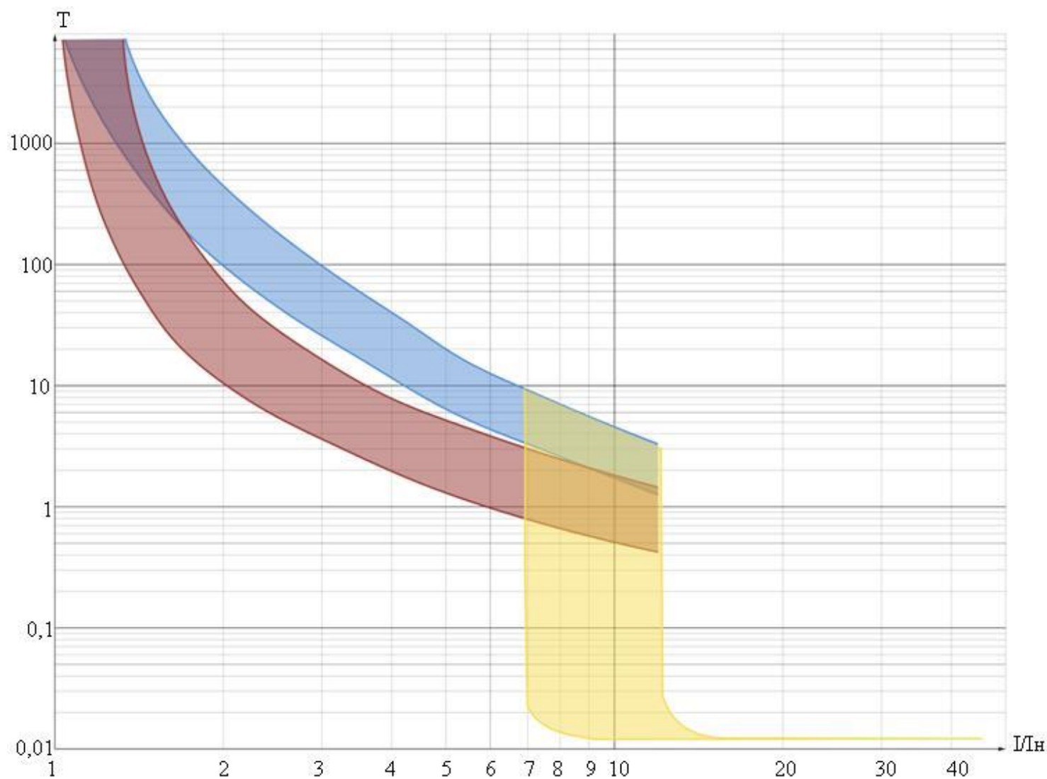
Рисунок Ж.7 - Время-токовые характеристики выключателя BA57-35 для номинальных токов тепловых максимальных расцепителей тока 63, 80 А
