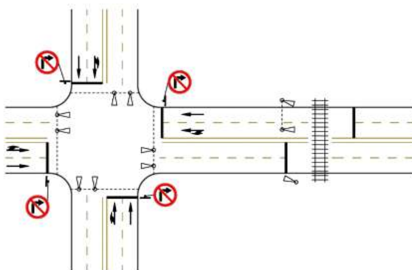
Рисунок К.4 - Схема размещения дополнительных светофоров
