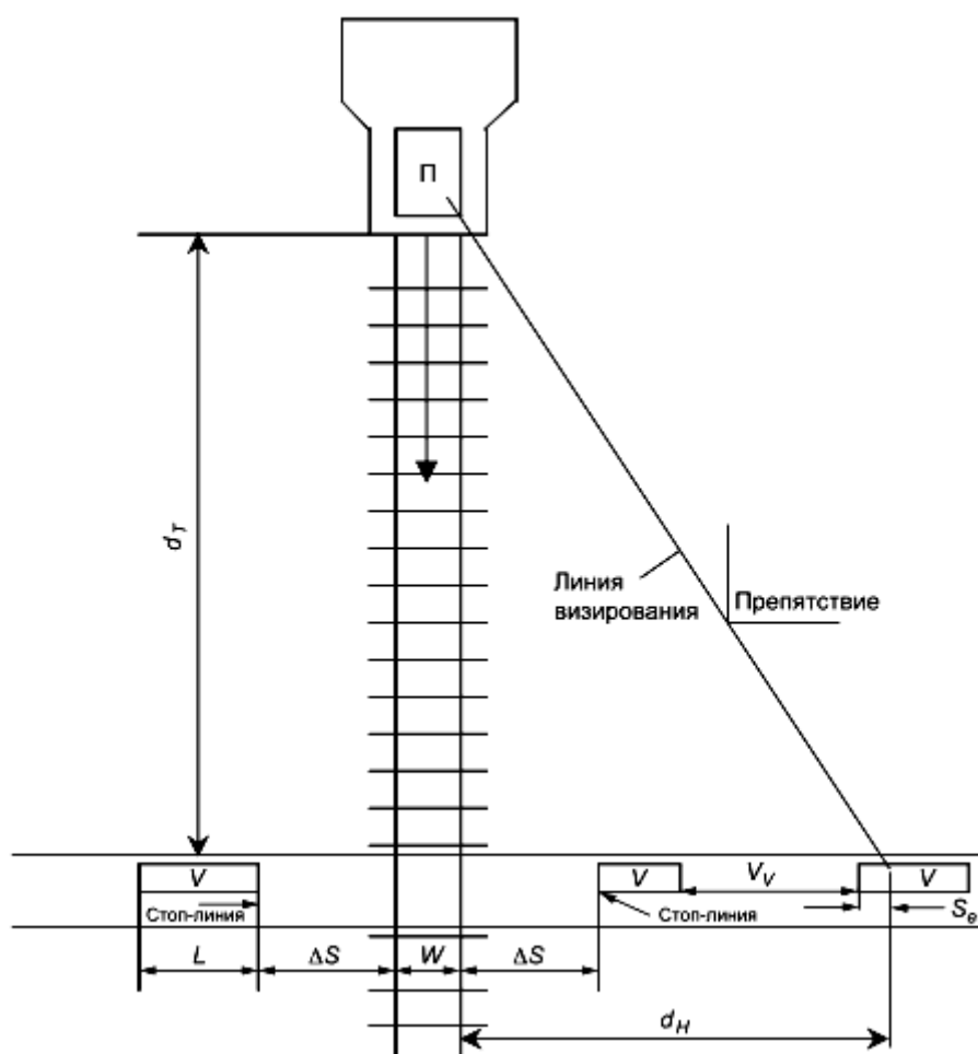
Рисунок К.1 - Схема определения расстояния видимости железнодорожного переезда (сигналов переездной сигнализации и шлагбаумов) вдоль автомобильной дороги d_H и расстояния видимости приближающегося к переезду поезда вдоль железнодорожных путей d_T
