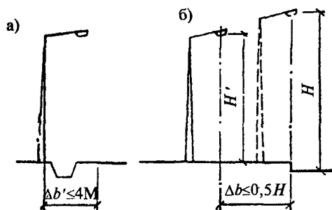
Рис. 5. Схемы допустимого расположения опор а — за кюветом; б — со смещением от проезжей части; H — допустимая высота установки светильника на границе проезжей части по условиям ограничения слепящего действия; \Delta b — смещение светильника от границы проезжей части; H' — допустимая высота смещенного светильника; \Delta b' — расстояние от опоры до границы проезжей части
