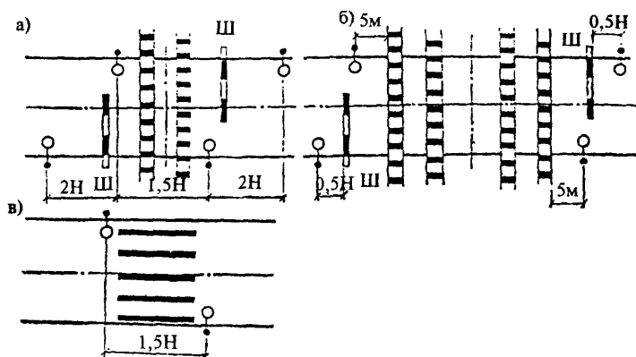
Рис. 3. Схемы размещения светильников
