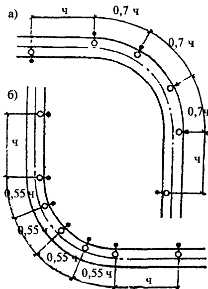
Рис. 2. Схемы размещения светильников на закруглениях улиц и дорог
