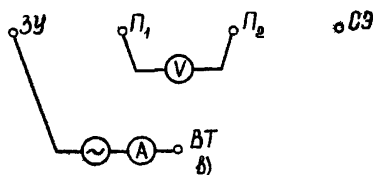
Рис. 5. Схемы трех последовательно используемых вариантов включения измерительных приборов при измерениях по методу СибНИИЗ (см. рис. 4)
