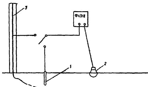
Рис. ПЗ.1. Схема измерения электрохимического окислительно-восстановительного потенциала:
