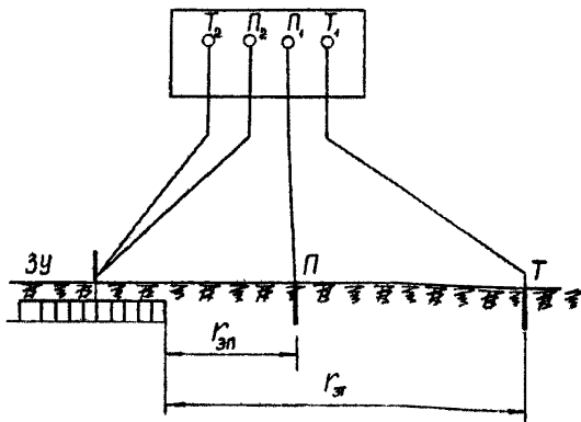
Рис. 2. Принципиальная схема измерений сопротивления ЗУ:
