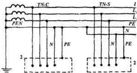
Рис. 10.4. Система TN-C-S
