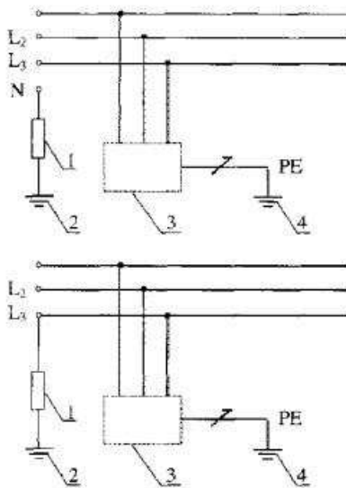
Рис. 1.5. Система IT
