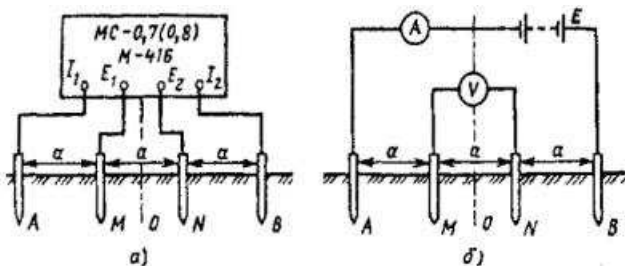
Рис. 11.1. Схема для определения удельного сопротивления грунта:
