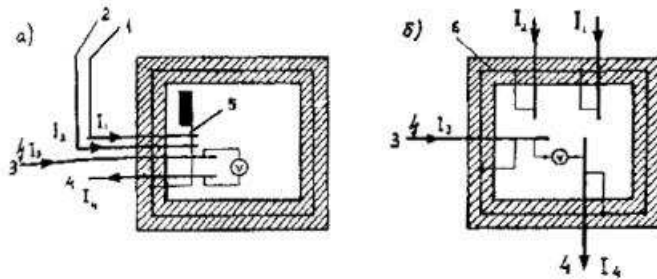
Рис. 2.1.7. Схемы ввода в здание металлических подземных коммуникаций:
