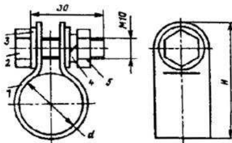
Рис. 7.10. Зажим типа ЗБХ:
