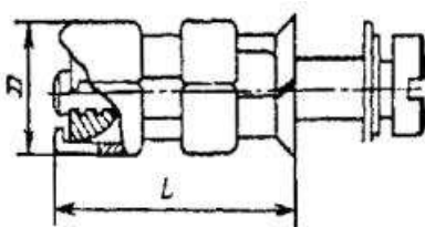
Рис. 7.2. Дюбель с распорной гайкой
