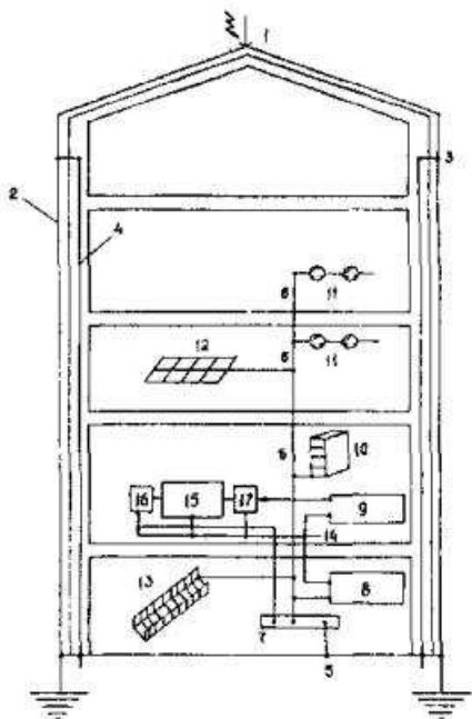
Рис. 2.1.4. Заземляющее устройство здания
