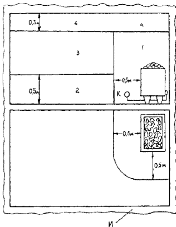
Рис. 10.10. Температурные зоны
