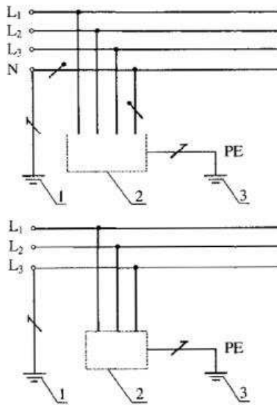
Рис. 1.4. Система TT
