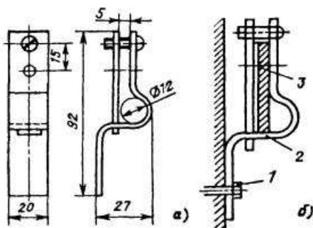
Рис. 7.1. Держатель шин заземления:
