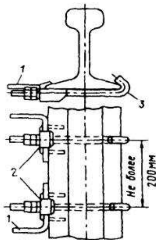
Рис. 8.3. Присоединение к тяговому рельсу проводников защитного заземления:
