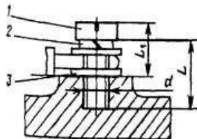
Рис. 7.6. Зажим типа ЗВ:
