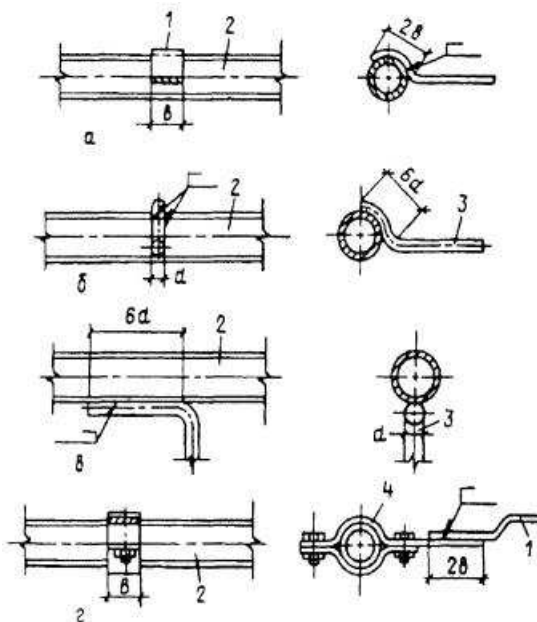
Рис. 8.8. Присоединение заземляющего проводника к трубопроводу сваркой ( a - e ) и с помощью хомута ( з ):
