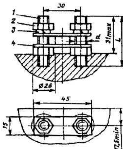
Рис. 7.8. Зажим типа ЗШ2П:
