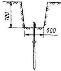
Рис. 8.4. Установка вертикальных заземлителей
