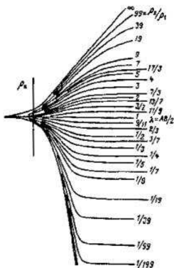
Рис. 11.2. Палетка ВЭЗ
