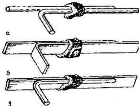
Рис. 8.10. Ответвления стальных заземляющих проводников, выполненные термитной сваркой
