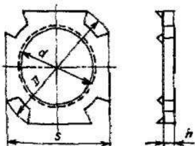
Рис. 7.13. Заземляющая установочная гайка
