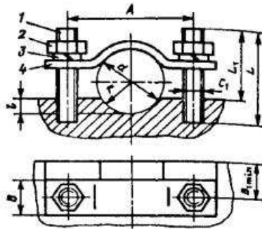
Рис. 7.8. Зажим типа ЗШ2С:
