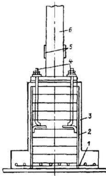
Рис. 8.2. Соединение металлической колонны с арматурой железобетонного фундамента:
