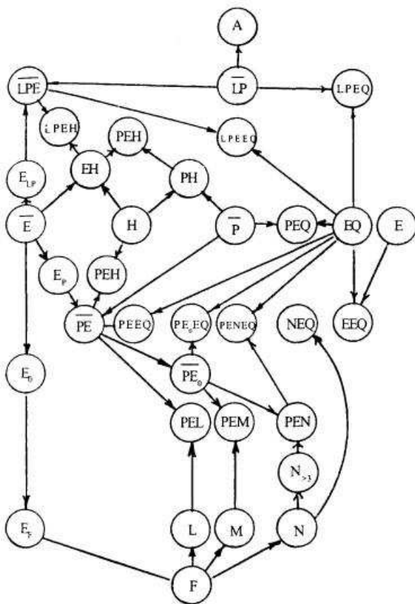
Рис. 2.2.1.А Классификация проводников (структурная схема)
