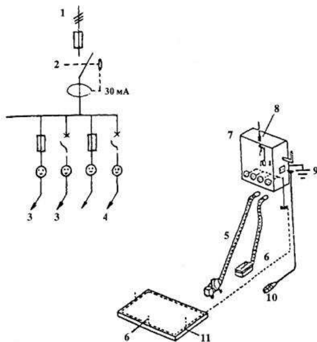
Рис. 10.5. Электроустановка, питающая строительную площадку небольших размеров
