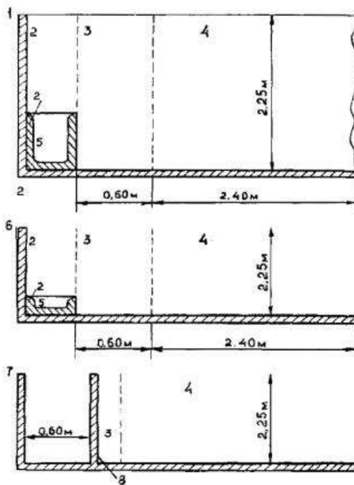
Рис. 10.9. В. Размеры зон (вертикальный разрез)
