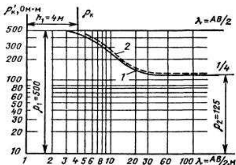
Рис. 11.2. Палетка ВЭЗ
