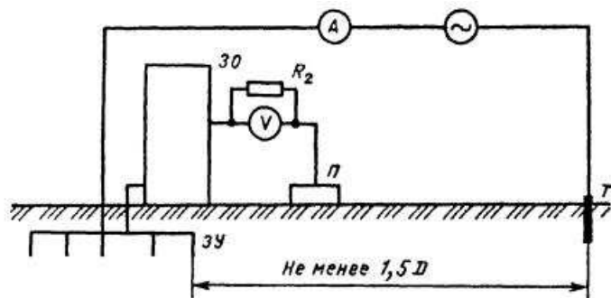
Рис. 11.8. Принципиальная схема измерения напряжения прикосновения по методу амперметра-вольтметра:
