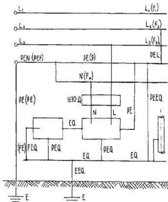
Рис. 2.2.2. Защитное и рабочее заземления в системе TN.
