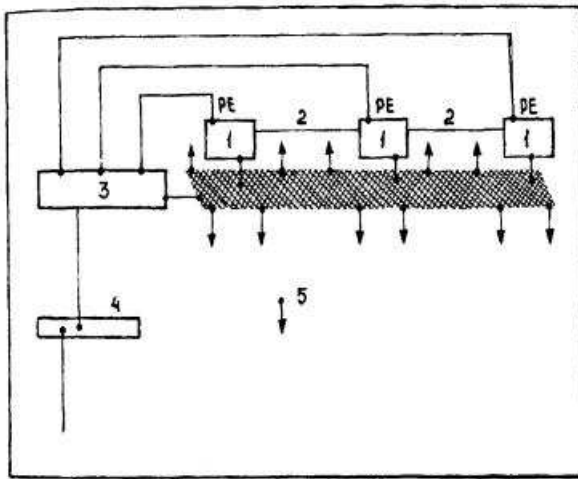
Рис. 2.2.7. Использование горизонтальных и вертикальных систем уравнивания потенциалов
