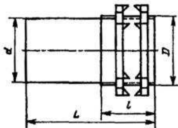
Рис. 7.14. Вводный патрубок
