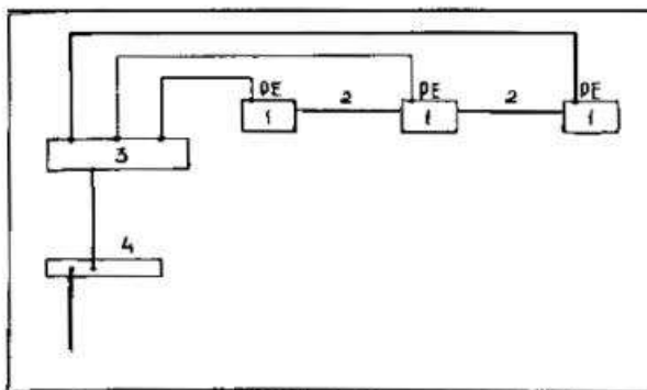
Рис. 2.2.5. Радиально соединенные защитные проводники
