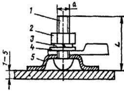
Рис. 7.7. Зажим типа ЗВП:
