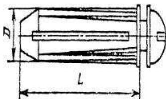
Рис. 7.3. Распорный капроновый дюбель
