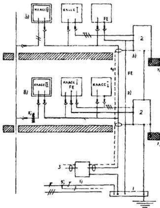
Рис. 2.1.3. Меры защиты электроустановок зданий от электромагнитных влияний:
