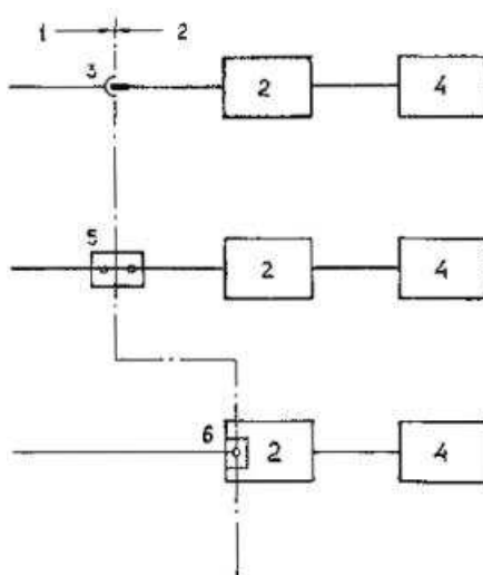
Рис. 2.2.3. Питающая электроустановка и информационно-технологическое оборудование
