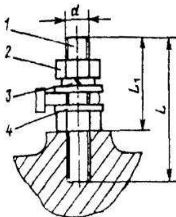
Рис. 7.4. Зажим типа ЗШ:
