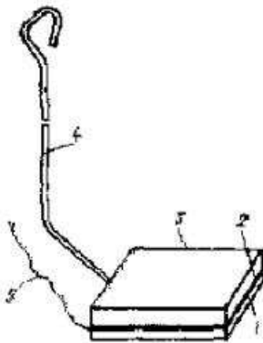
Рис. 11.10. Потенциальный электрод, имитирующий две ступни человека:
