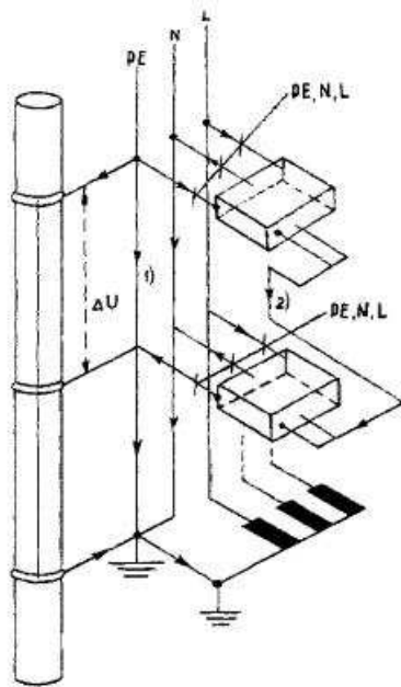
Рис. 2.1.6. Система питания электроустановок многоэтажного здания TN-S
