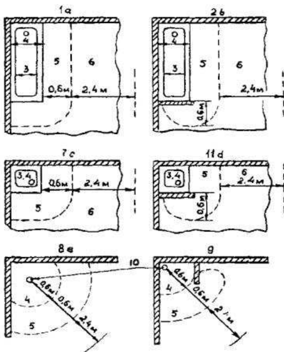
Рис. 10.9.А. Размеры зон (план)
