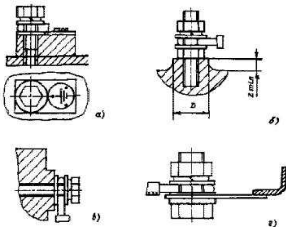
Рис. 7.12. Варианты установки зажимов:
