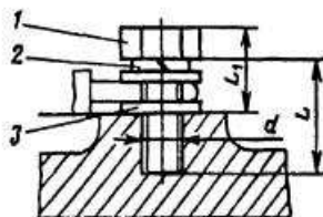
Рис. 7.5. Зажим типа ЗБ:
