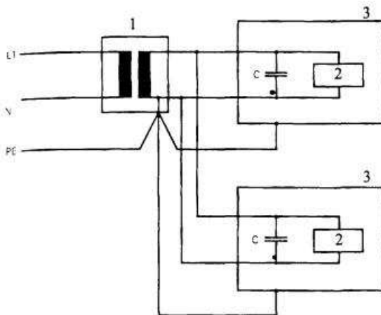
Рис. 2.2.8. Питание ИТО через разделяющий трансформатор
