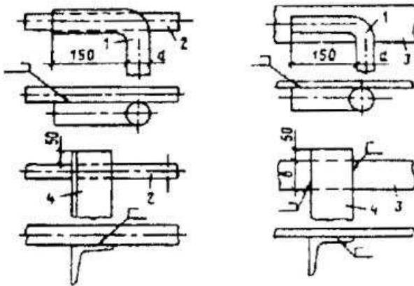
Рис. 8.6. Соединение заземляющих проводников с вертикальными заземлителями:
