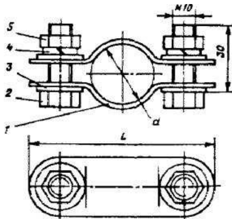
Рис. 7.11. Зажим типа ЗБ2:
