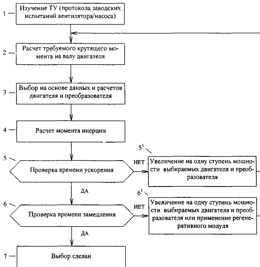
Рис. 2 Схема алгоритма выбора преобразователя частоты и двигателя для вентилятора/насоса
