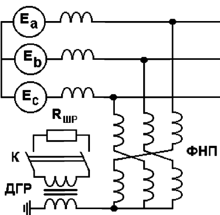
Рисунок 7.2 – Схема подключения регулируемого дугогасящего реактора с шунтирующим резистором
